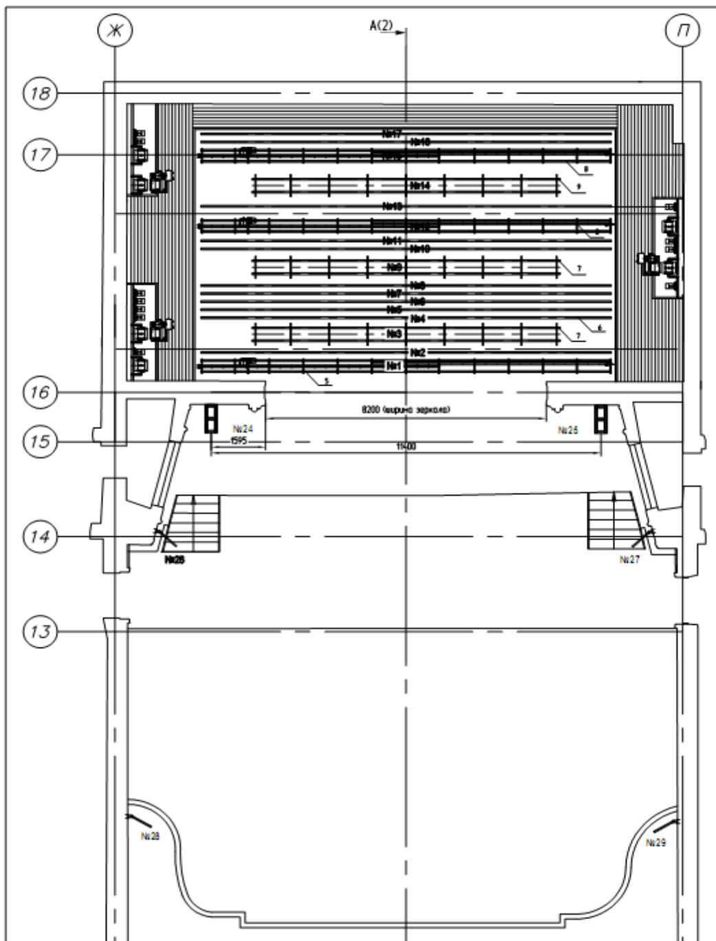
План зрительного зала и планшета сцены (1:75)
